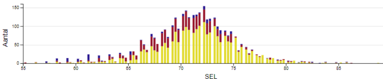
Figuur 5.4: Verdeling geluidniveaus van vliegtuigpassages oktober (maandgemiddeld).
