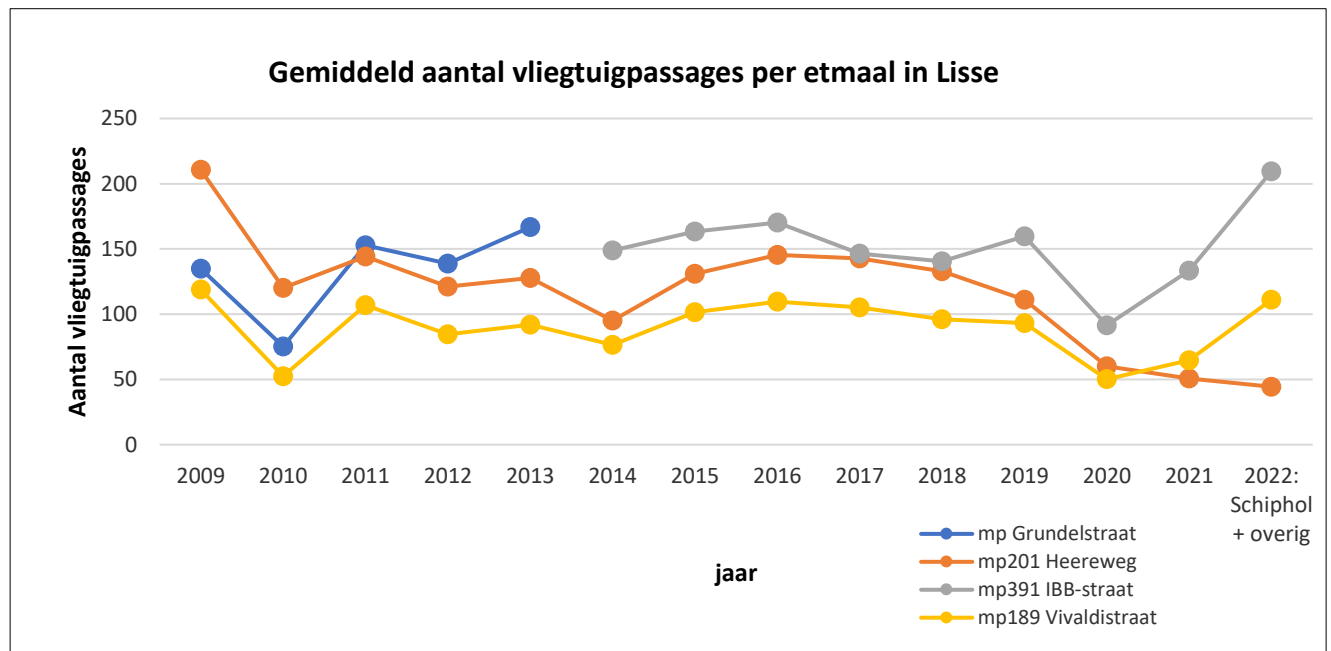
Figuur 7.2: Trend gemiddeld aantal vliegtuigpassages per etmaal in Lisse. NB: meetpost Grondelstraat is medio 2014 vervangen door een meetpost Ina Boudier-Bakkerstraat (IBB-straat).
