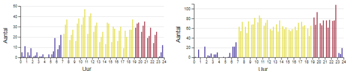
Figuur 5.2: Verdeling vliegtuigpassages over het etmaal, maandgemiddeld in Katwijk (links: september 2022, rechts: oktober 2022).
