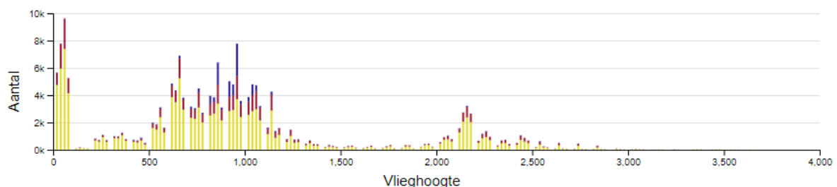
Figuur 6.6: Aantal passages per vlieghoogte.
