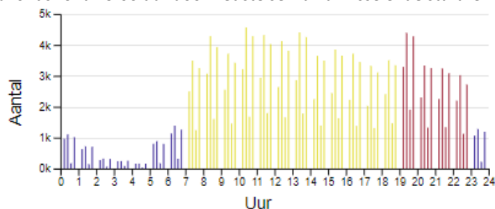
Figuur 10.3: Verdeling vliegtuigpassages over het etmaal (jaargemiddeld).
