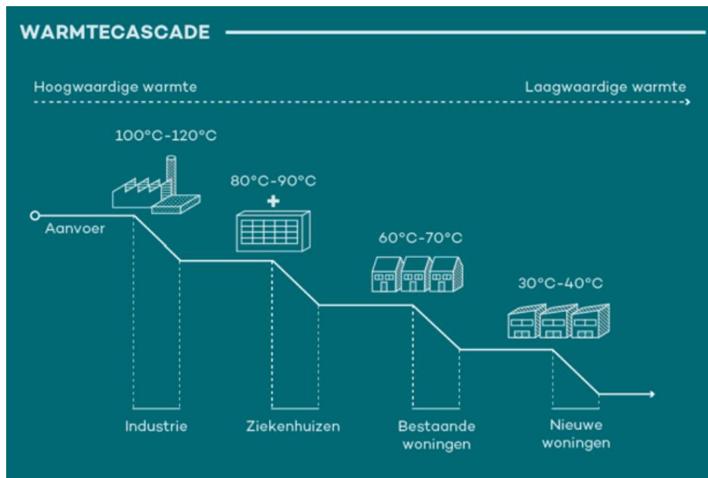
Figuur: 5.1: warmtecascade.
